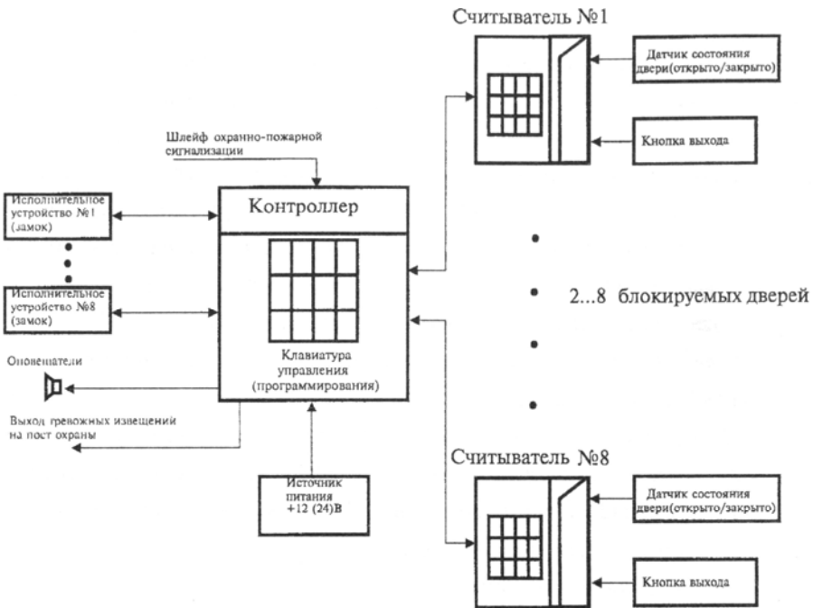
Рисунок 2 – Оборудование СКУД объекта с несколькими дверьми
