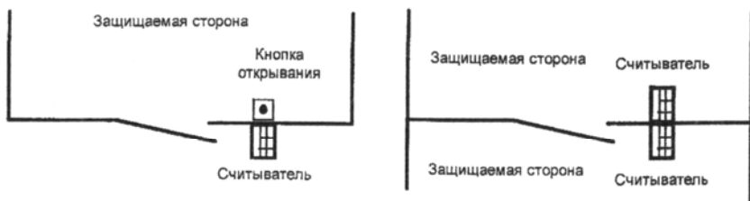
Размещение считывателей на стене
