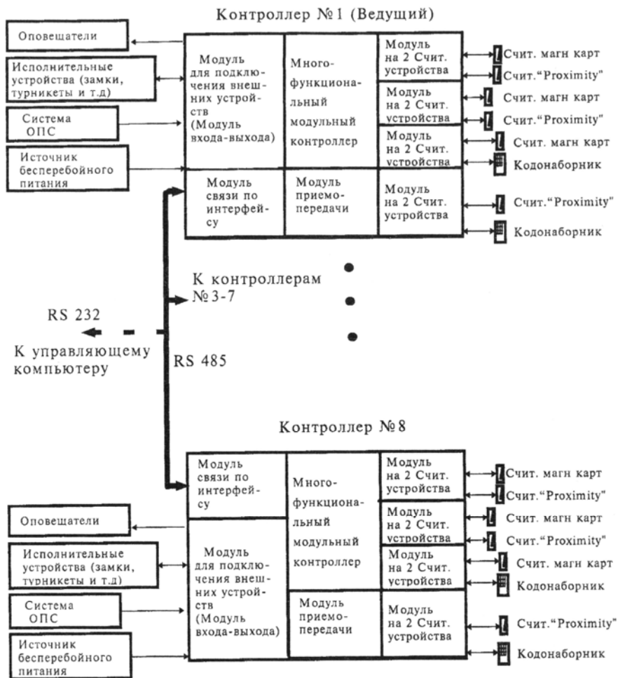
Рисунок 3 – Примерная структурная схема построения сетевой СКУД
